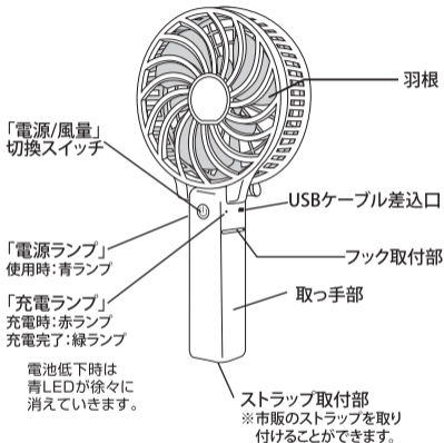
<本体正面>
